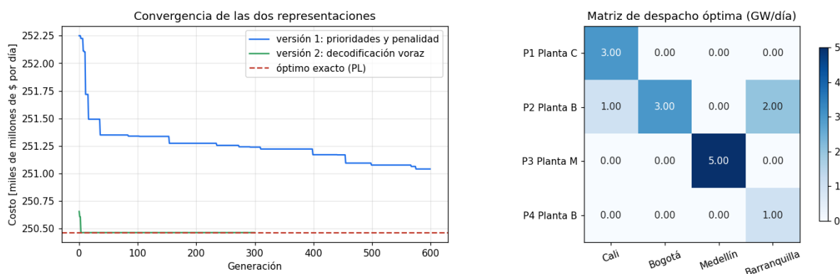
Figura 4. A la izquierda, convergencia de las dos representaciones frente al óptimo exacto. A la derecha, matriz de despacho obtenida con la decodificación voraz.
